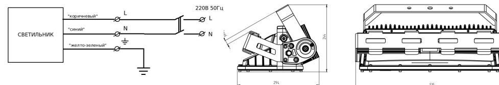
Рисунок 1. Электрическая схема подключения.
