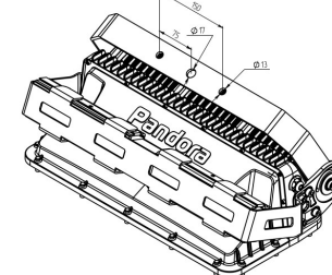
Рисунок 2. Габаритный чертёж
